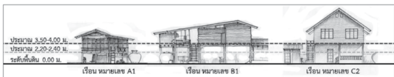
ภาพที่ 8 เปรียบเทียบความสูงของพื้นที่ 2 ของเรือนหมายเลข A1 B1 และ C2 (ที่มา: ผู้วิจัย)
